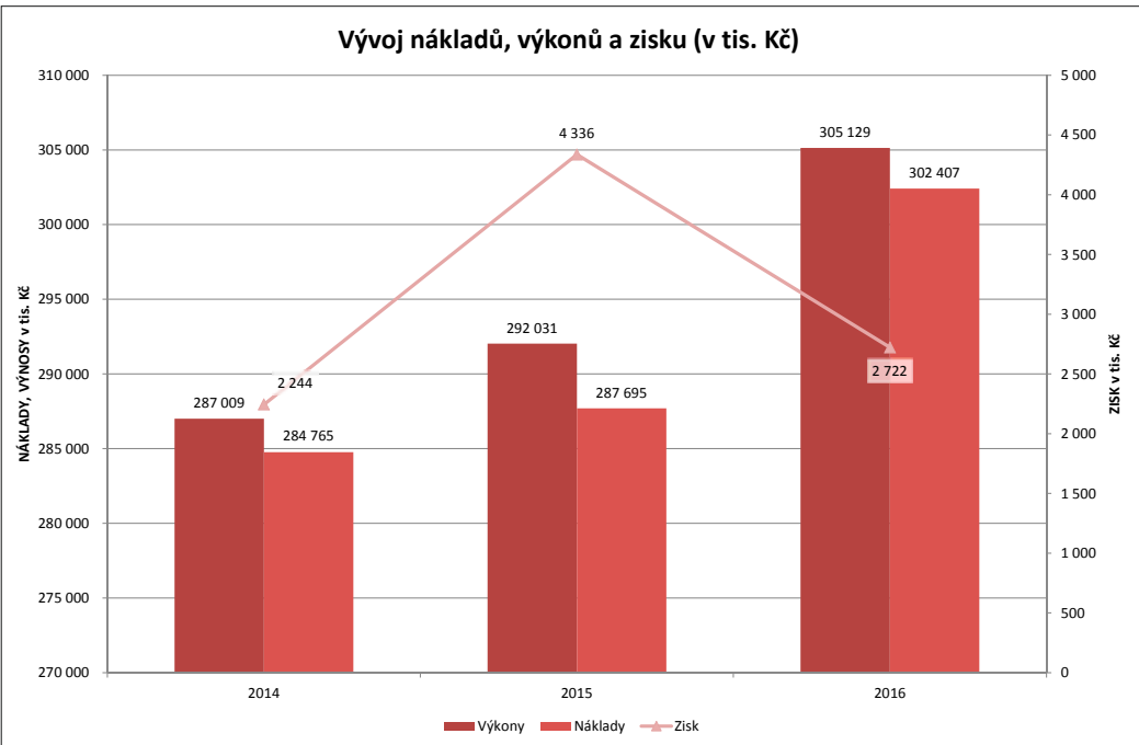
Graf č. 1 – Vývoj nákladů, výkonů a zisku v letech 2014 – 2016
